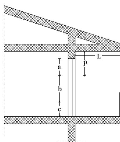
Schema esplicativo superficie illuminante utile
